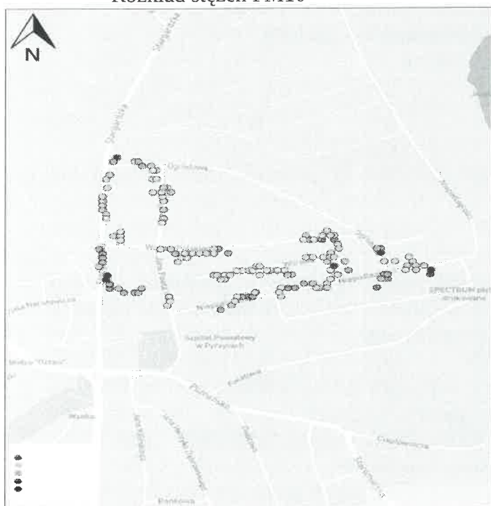
Rozkład stężeń PM 10
