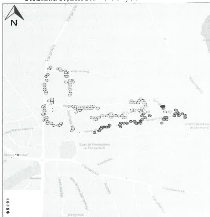
Rozkład stężeń formaldehydu
